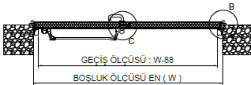
B-B KESİTİ
