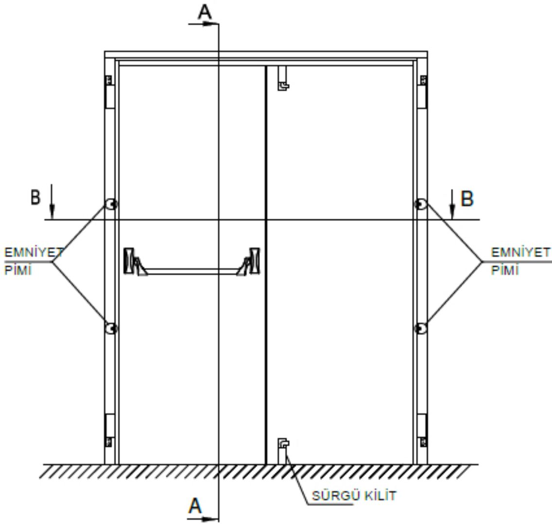
A-A KESİTİ
