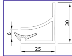
4 Çatı profili ve sıkıştırma contası
