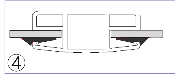
4 Çatı profili ve sıkıştırma contası
